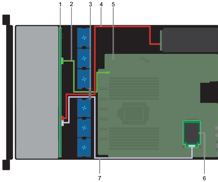
图 95: 电缆布线 — 12 x 3.5 英寸驱动器背板
