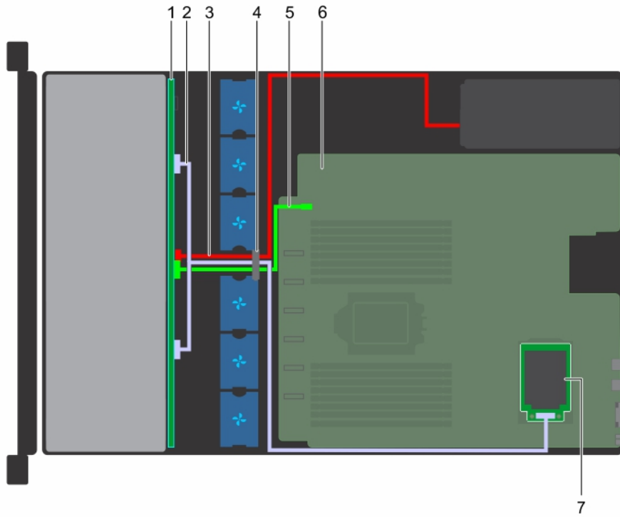
图 93: 电缆布线 — 8 x 3.5 英寸驱动器背板, 带 mini PERC 卡
