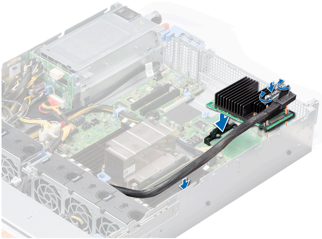
图 91: 安装 Mini PERC 卡
