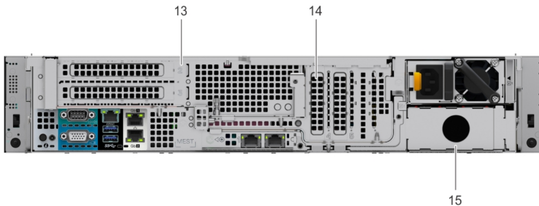
图 11: 提升板 1B 系统的背面板功能部件
