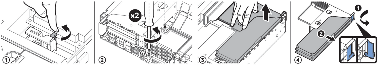
图 22: 提升板 1B 安装
