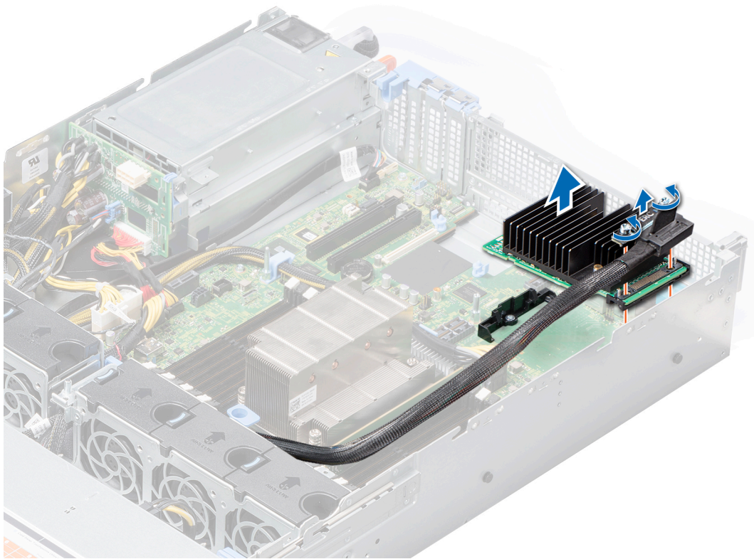
图 90: 卸下 Mini PERC 卡
