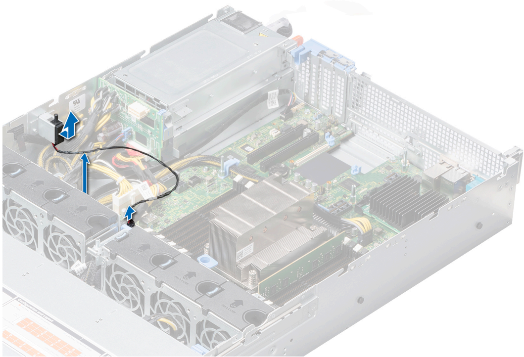
图 38: 卸下防盗开关
