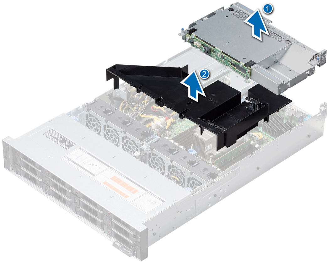
图 32: 卸下带背面驱动器固定框架的系统上的导流罩
