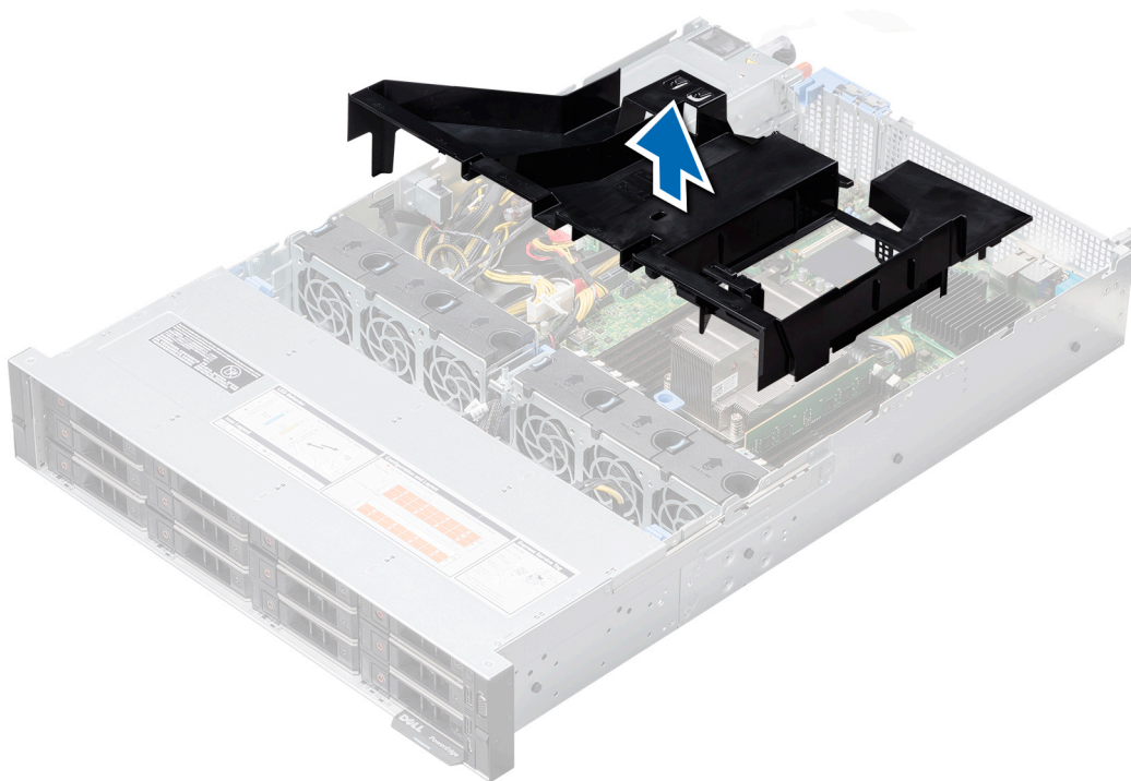
图 31: 卸下不带背面驱动器固定框架的系统上的导流罩
