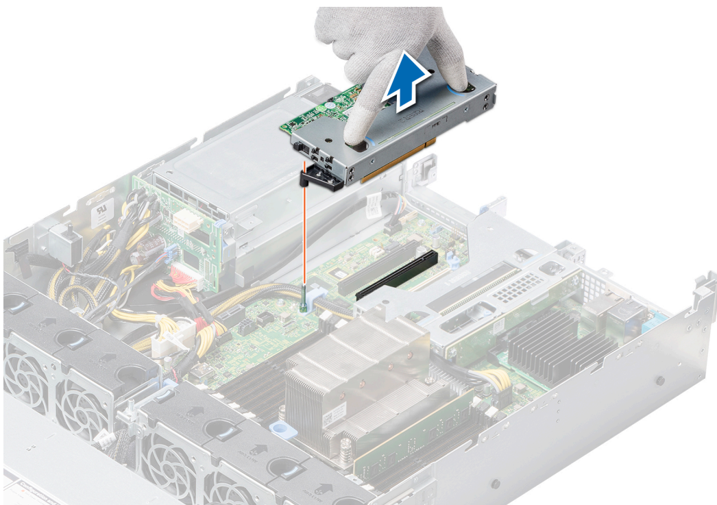
图 76: 卸下提升板 3A
