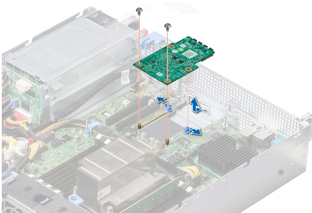
图 84: 卸下 LOM 提升卡
