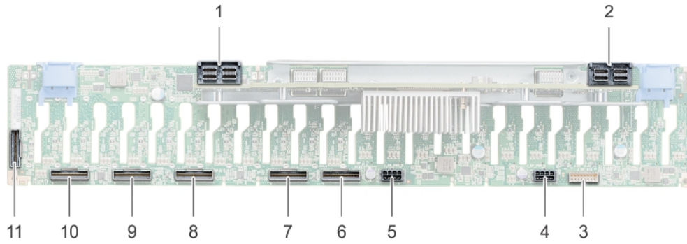
图 61: 24 x 2.5 英寸驱动器背板
