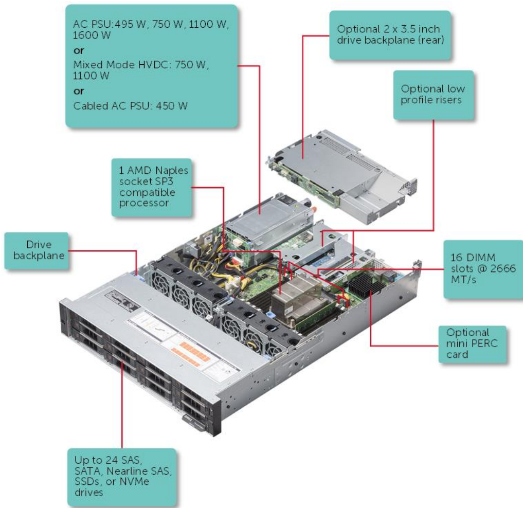
图 1: 带背面驱动器的 PowerEdge R7415 系统支持的配置
