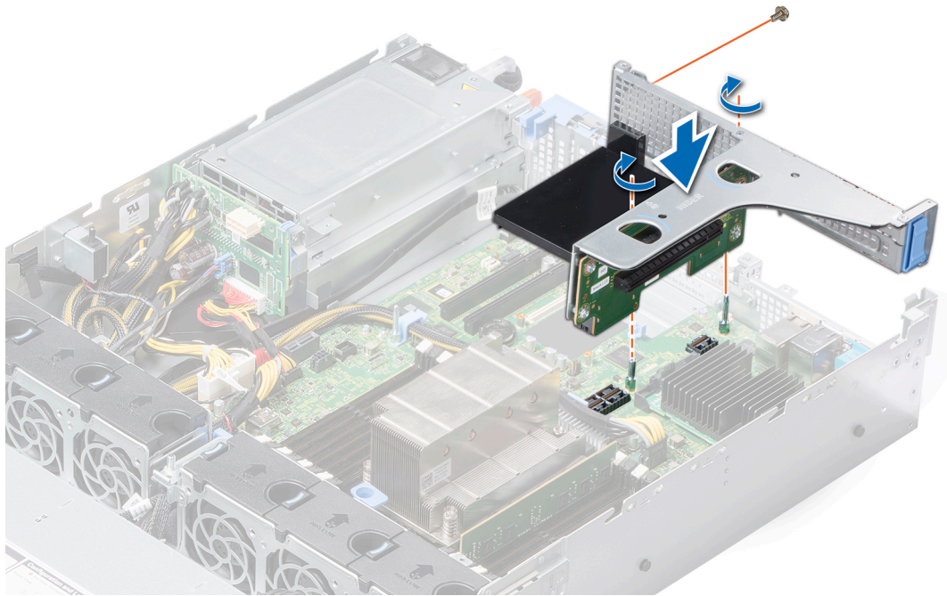
图 81: 安装提升板 1B
